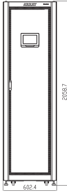
前视图
