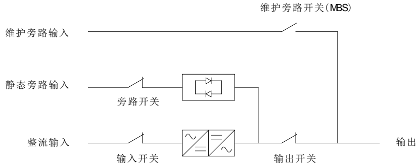
图 6-7: 维护旁路开关和 MBS 开关的正常位置
