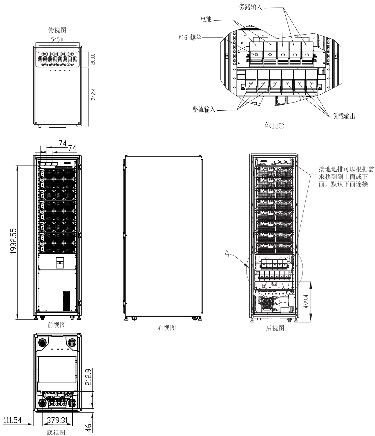
图 4-1: ARRAY 3A3 PT 25-200 kVA UPS 盖板 and 连接端子位置 (带内置电池版本)
