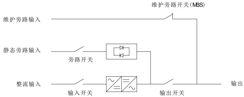
图 6-8: 维护旁路模式
