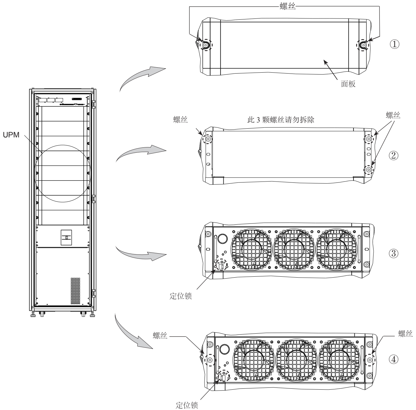
图 6-6: UPM 模块位置
