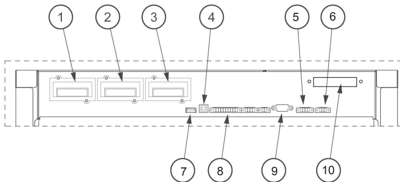
图 5-1：通信接口
