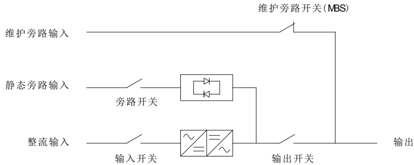
图 6-9: 维护旁路模式
