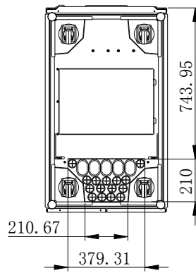
底视图
