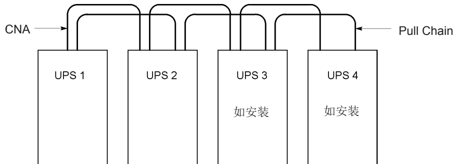
图 4-5: 并机 UPS 系统的 CAN 和 pull-chain 的简化配线
