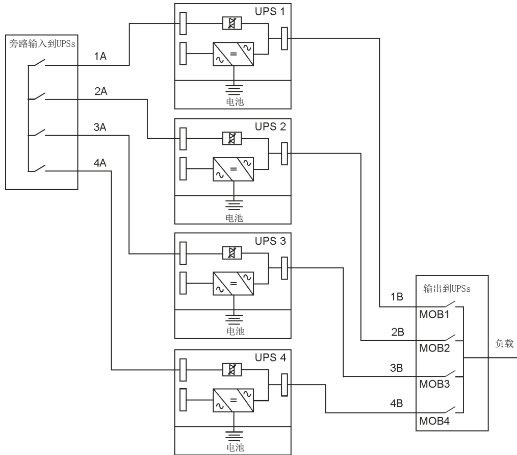
图 4-3: 并机 UPS 系统的原理
