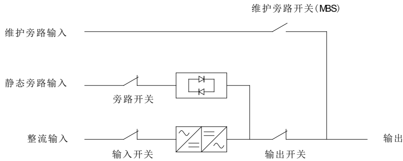
图 6-10: 正常模式
