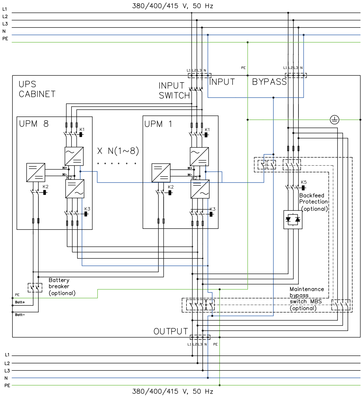
图 2-2: ARRAY 3A3 PT 25-200 kVA UPS 结构图
