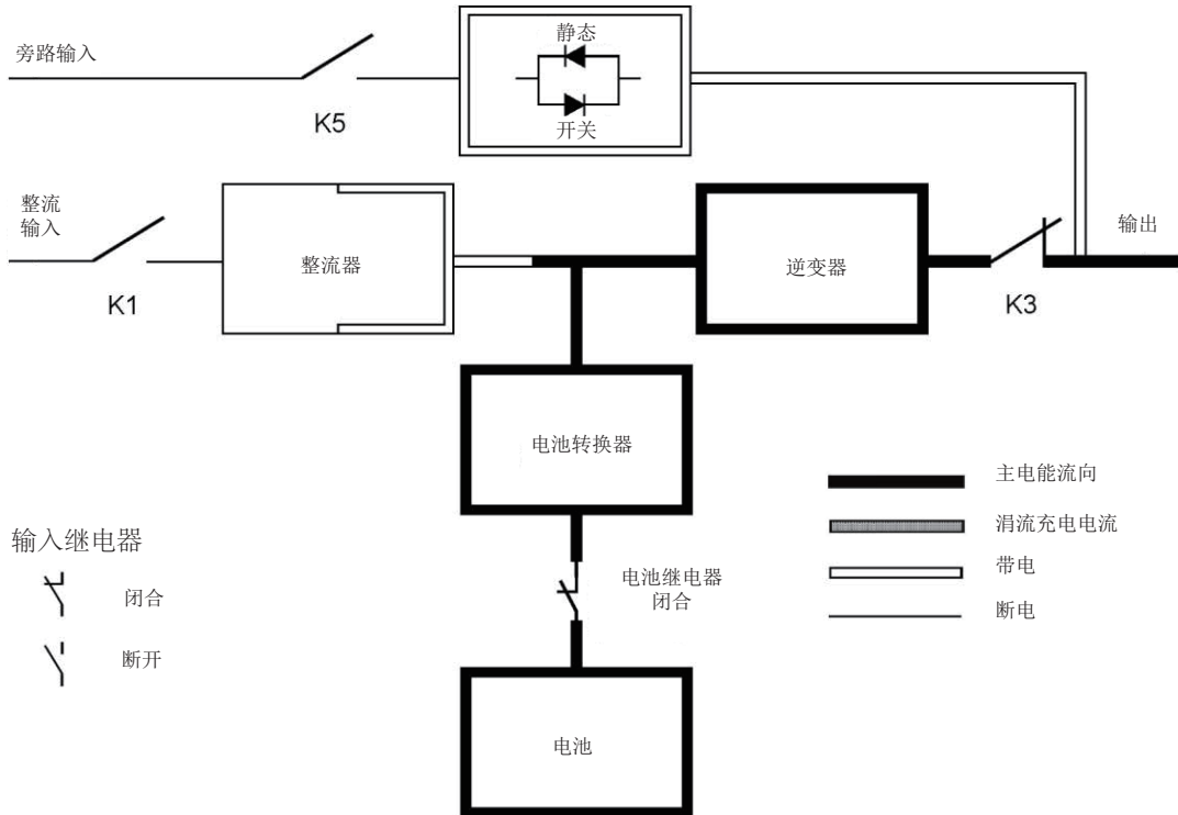
图 2-6：电池模式下电能通过 UPS 的路径
