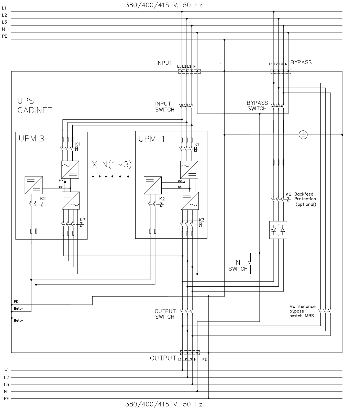
图 2-2: ARRAY 3A3 PT 25-75 kVA UPS 不带内置电池版本结构图
