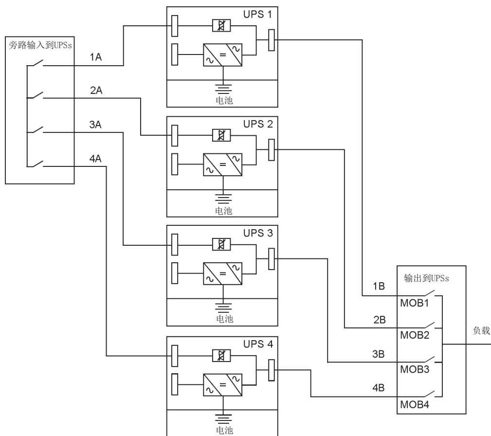
图 4-7: 并机 UPS 系统的原理
