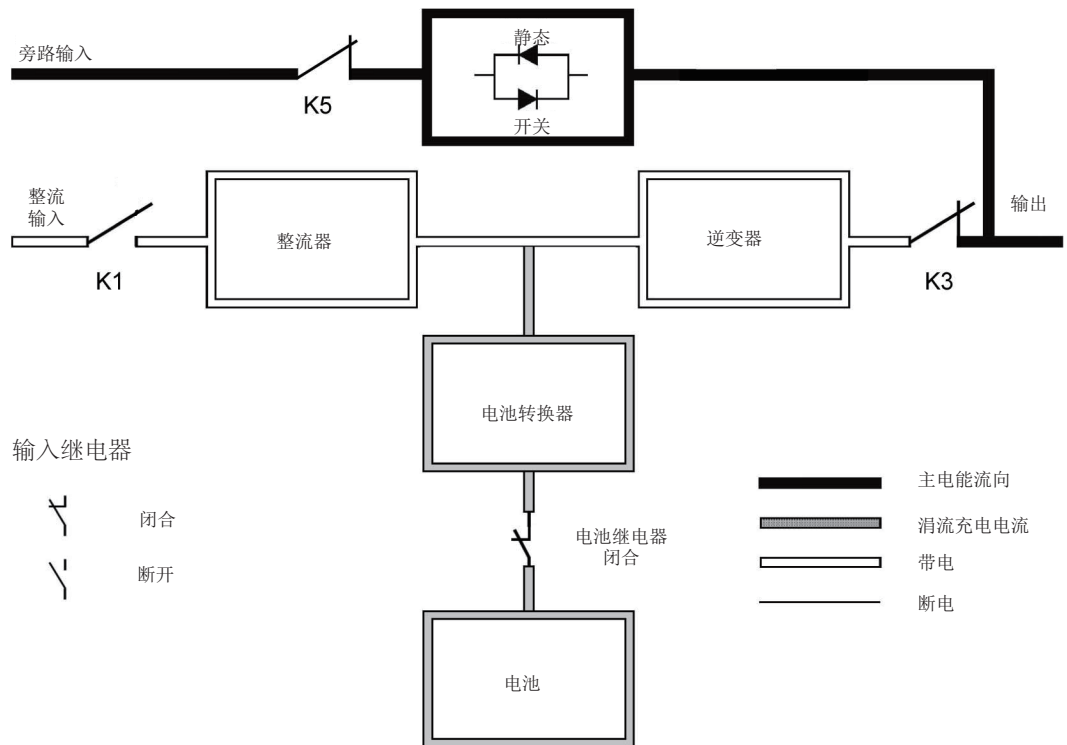
图 2-5: ECO 模式下电能通过 UPS 的路径
