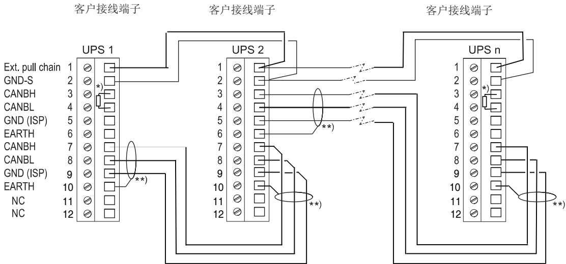
图 4-11: 不带 MOBs 的并机 UPS 的 CAN 和 Pull-chain 的配线
