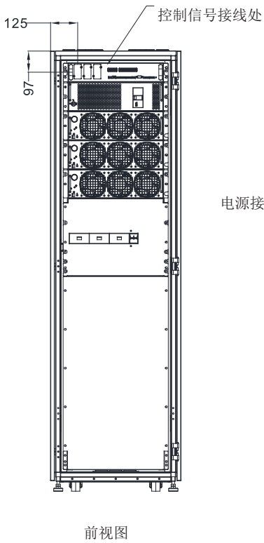
图 4-2: ARRAY 3A3 PT 25-75 kVA UPS 盖板和连接端子位置 (不带内置电池版本)
