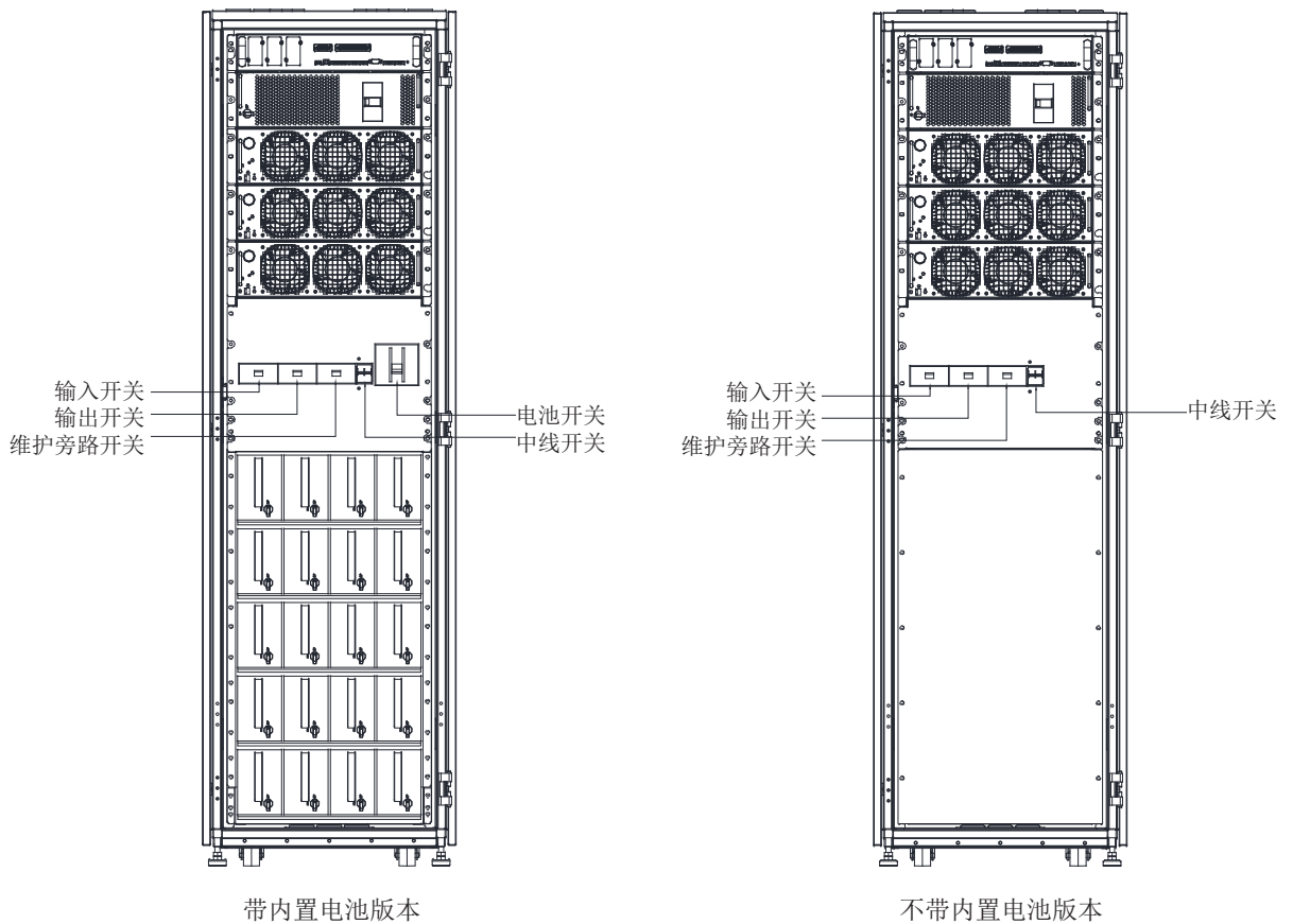
图 6-1: UPS 开关位置
