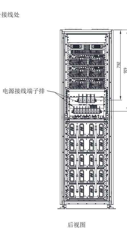
图 4-2: ARRAY 3A3 PT 25-75 kVA UPS 盖板和连接端子位置 (不带内置电池版本)
