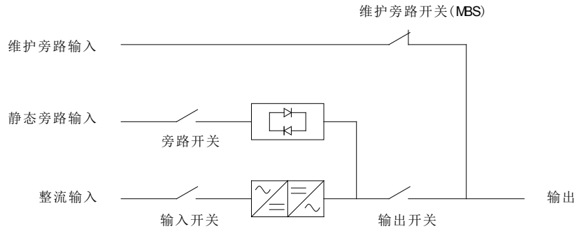
图 6-10: 维护旁路模式
