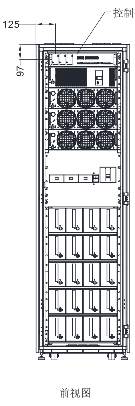
图 4-1: ARRAY 3A3 PT 25-75 kVA UPS 盖板和连接端子位置 (带内置电池版本)
