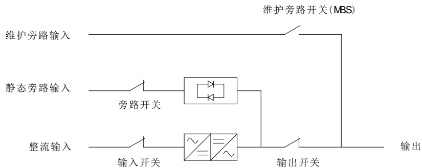
图 6-11: 正常模式
