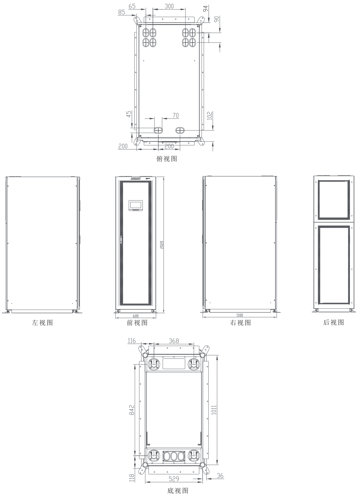
图 3-2: ARRAY 3A3 PT 25-75 kVA UPS 尺寸
