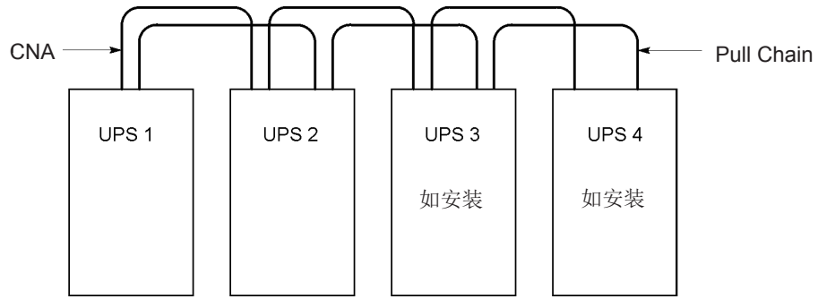
图 4-9: 并机 UPS 系统的 CAN 和 pull-chain 的简化配线
