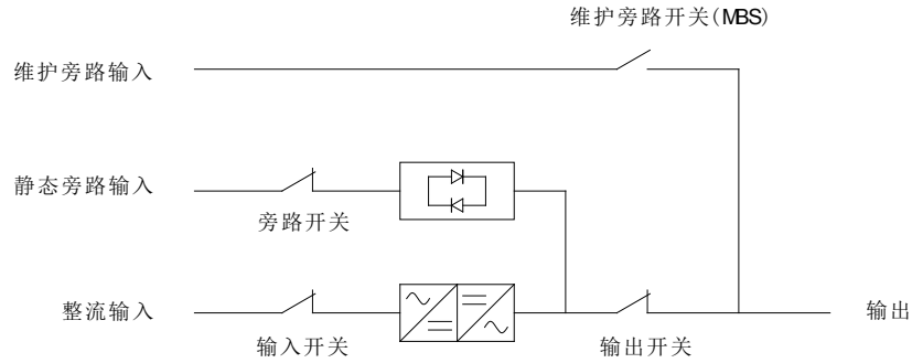
图 6-8: 维护旁路开关和 MBS 开关的正常位置
