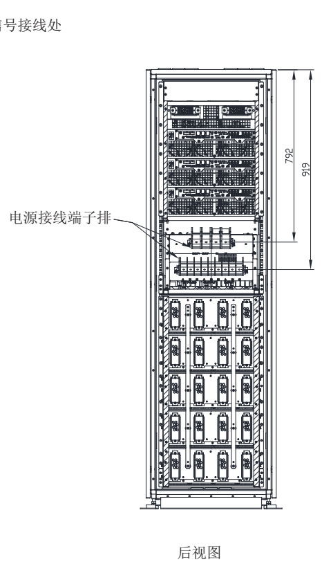
图 4-1: ARRAY 3A3 PT 25-75 kVA UPS 盖板和连接端子位置 (带内置电池版本)
