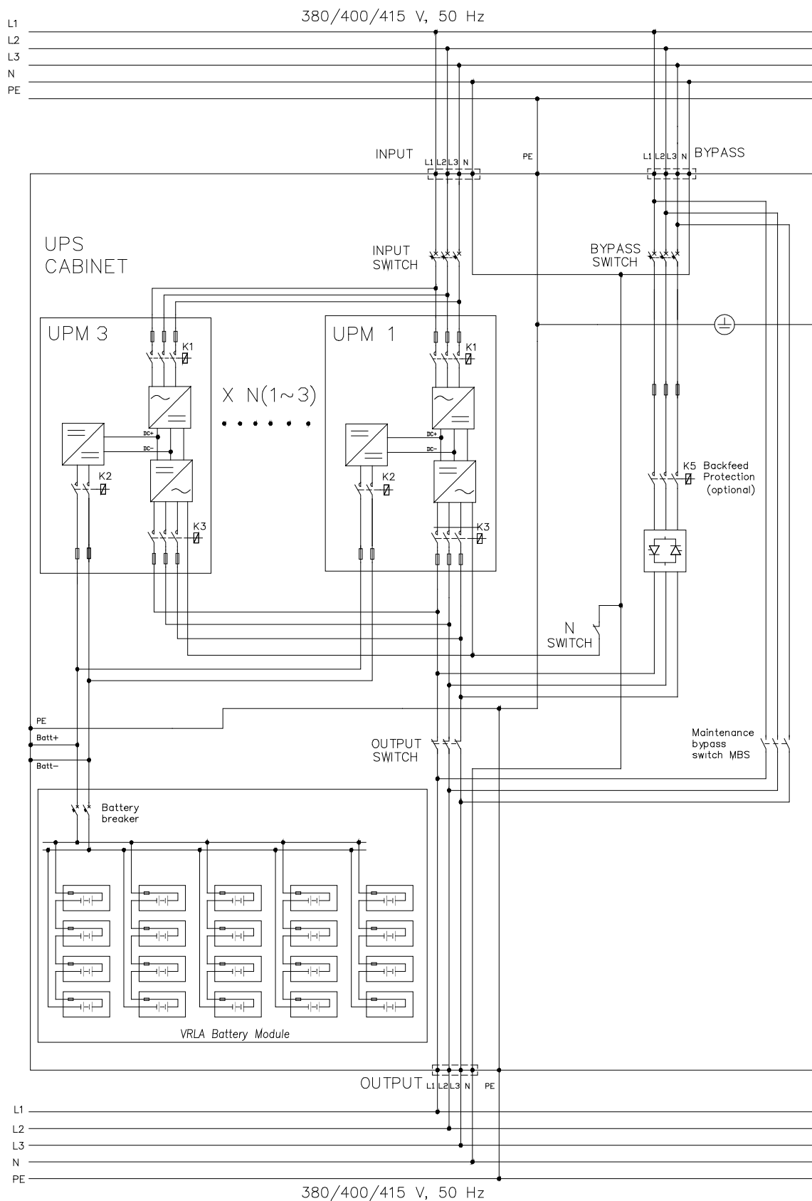
图 2-3: ARRAY 3A3 PT 25-75 kVA UPS 带内置电池版本结构图
