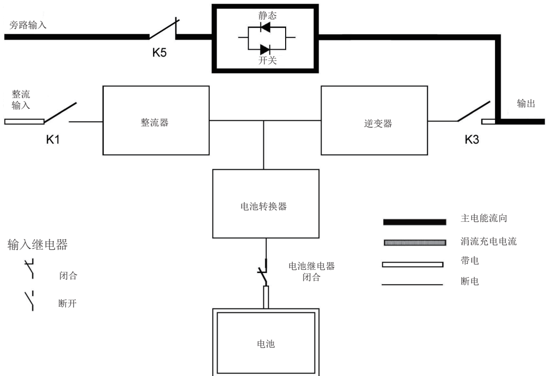
图 2-7：旁路模式电能通过 UPS 的路径
