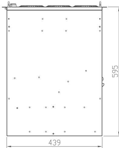
顶视图
