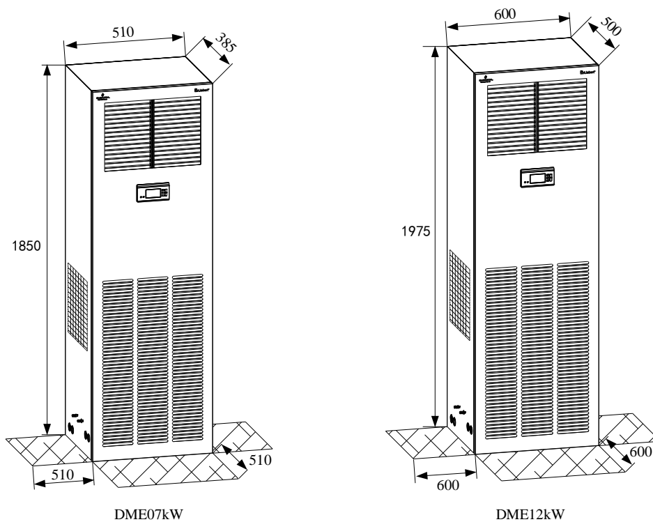
图2-3 室内机外形尺寸图（单位：mm）
