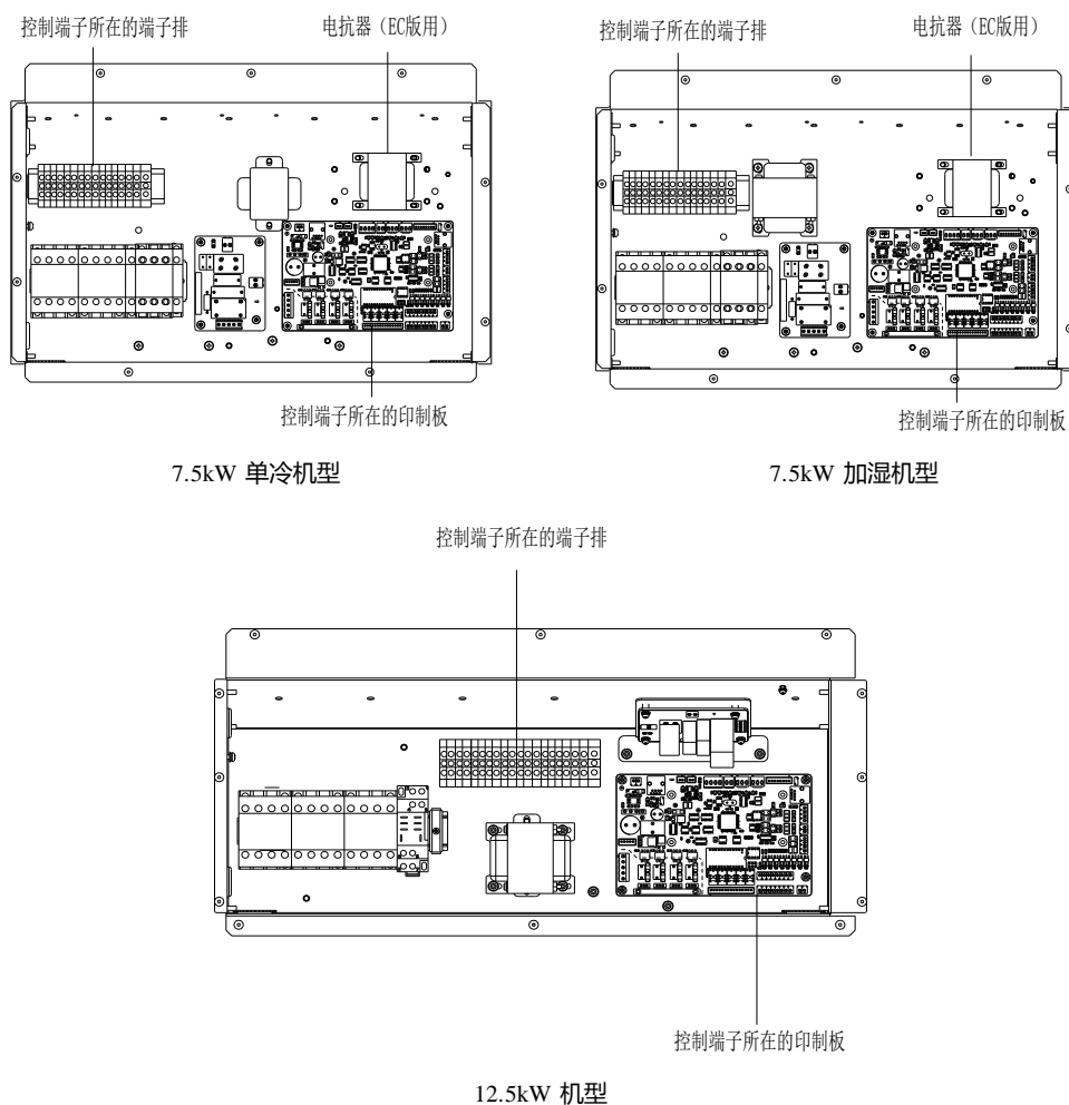
图3-5 控制端子位置
