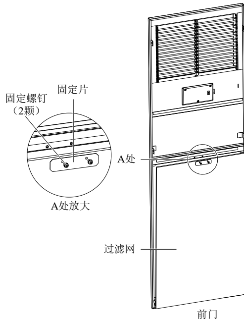
图6-1 取出前门过滤网
