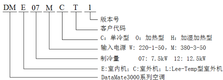
图1-1 型号说明
