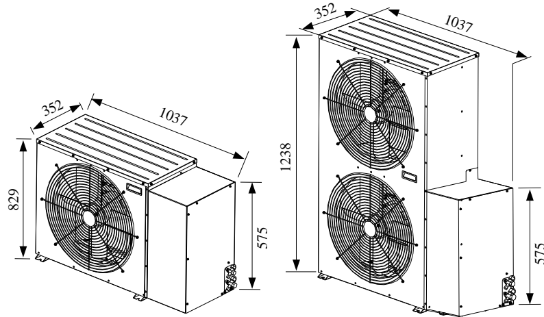
图2-5 Lee-Temp 型室外机外形尺寸图（单位：mm）
