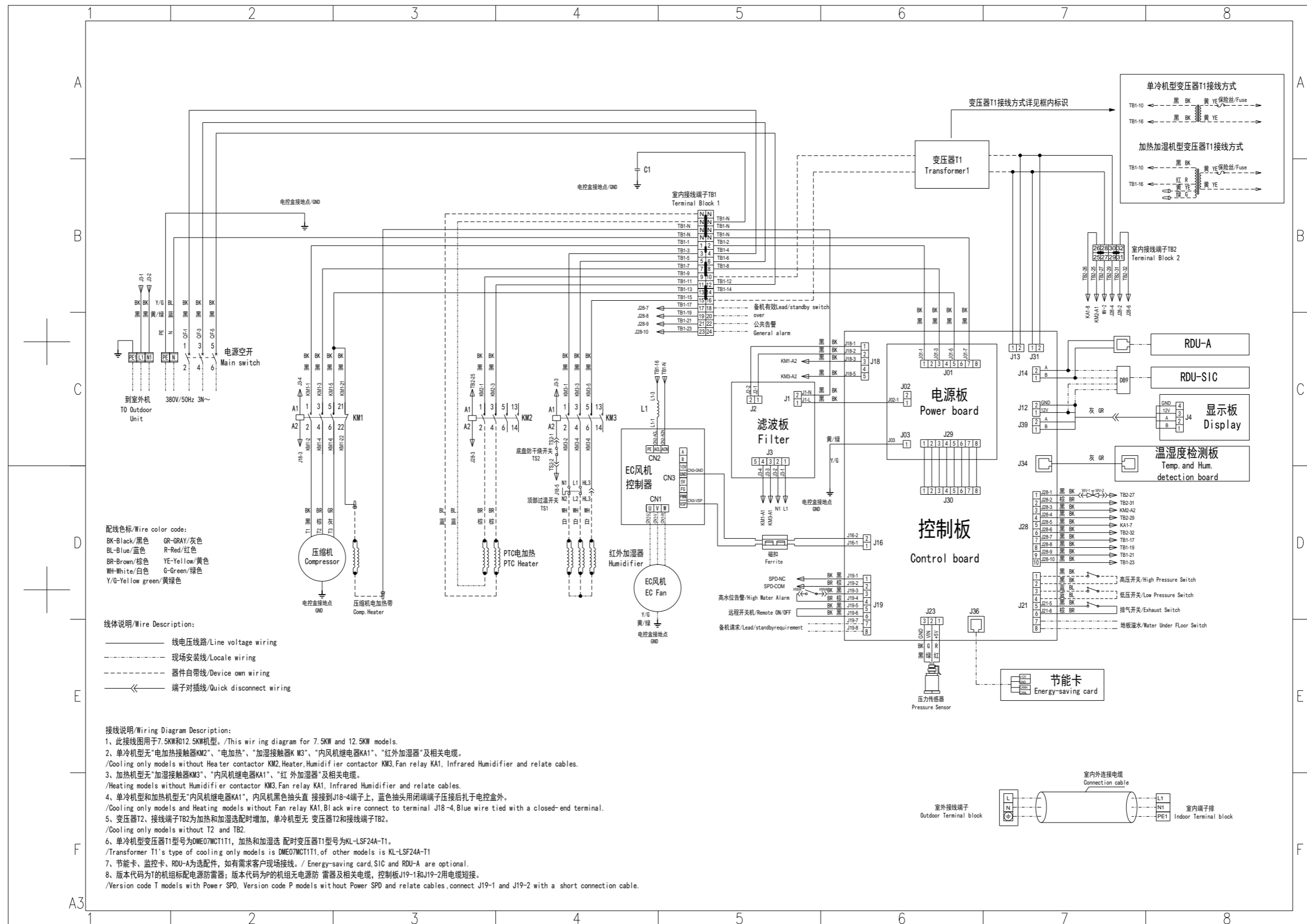
EC 风机版机组原理图
