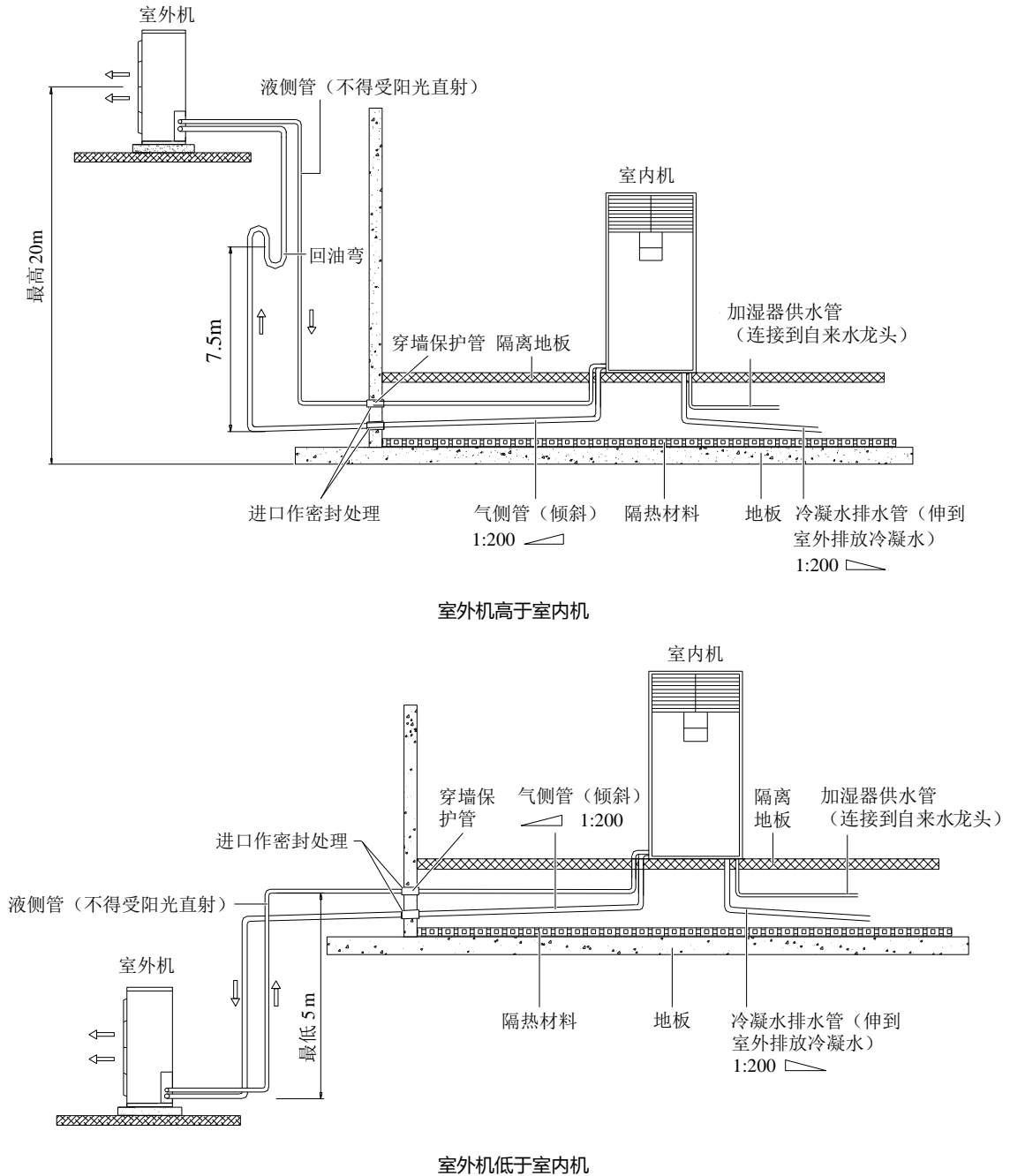
图2-2 安装示意图
