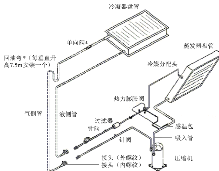
图2-1 总体布局图
