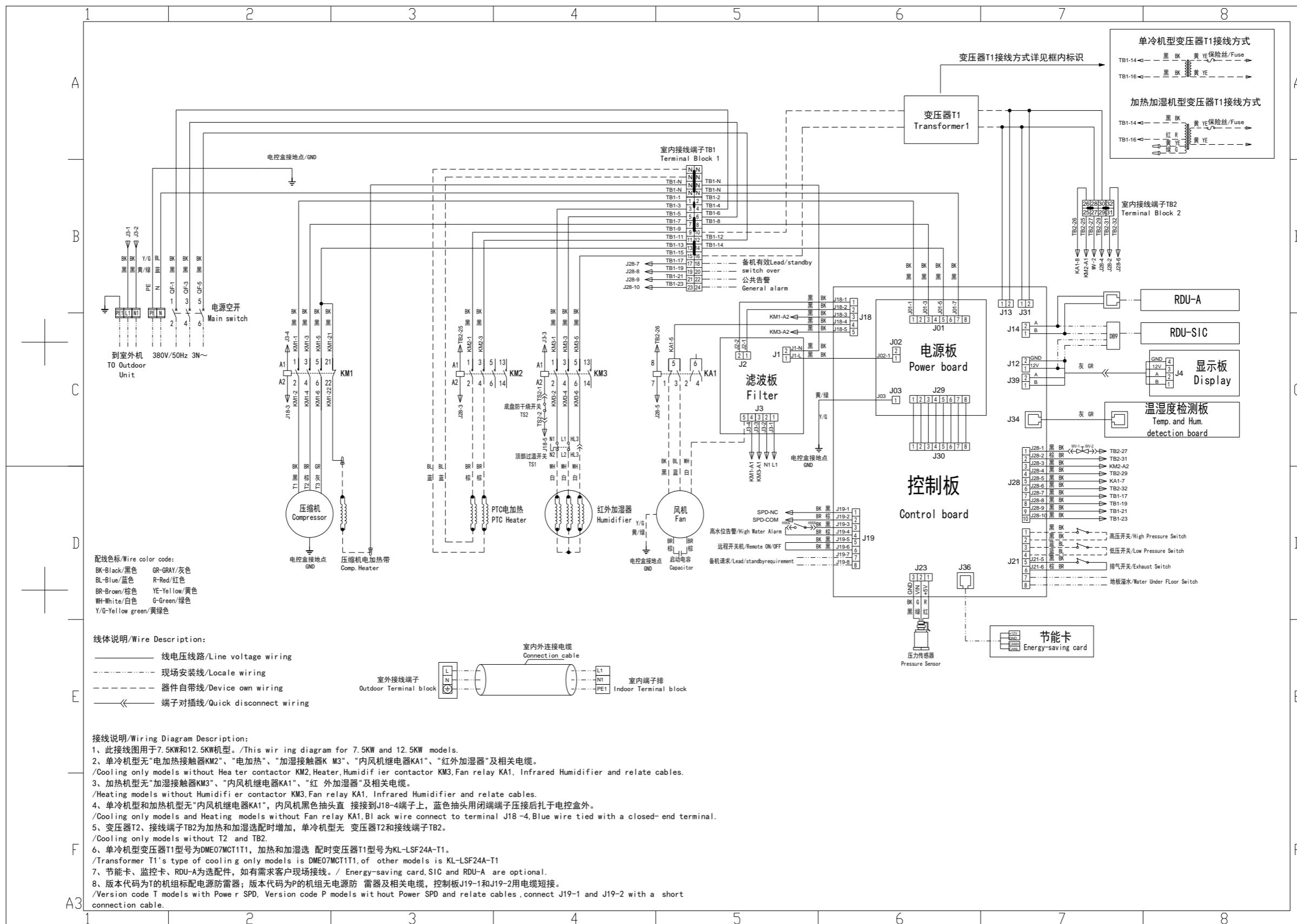
AC 风机版机组原理图
