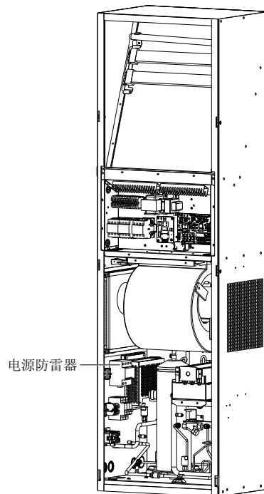
图6-5 电源防雷器位置
