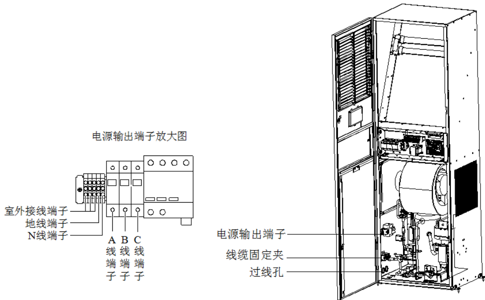
图3-2 室内机输入输出电源接线
