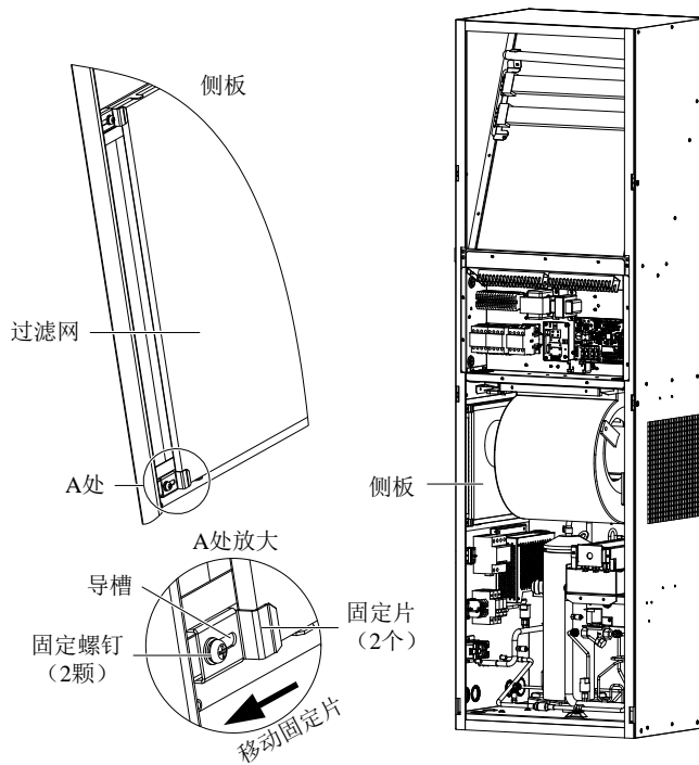
图6-2 取出侧板过滤网
