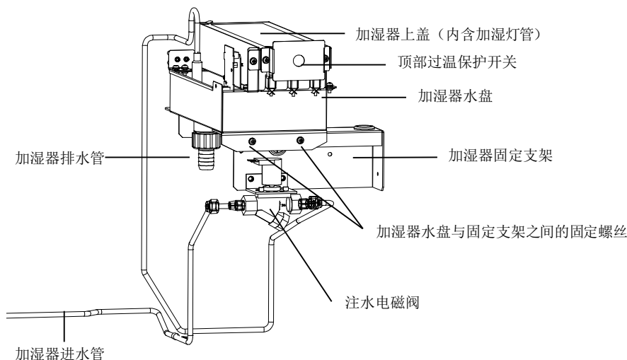
图6-3 加湿器
