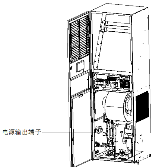
图3-1 室内机电源接线位置
